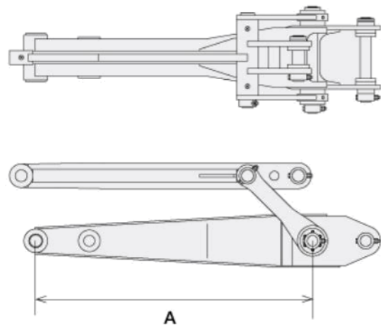
■エクステンションアーム 寸法図
