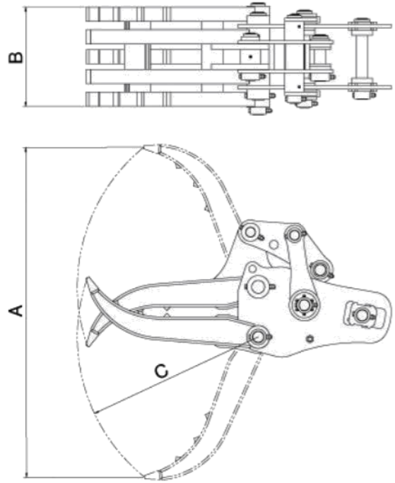
■グラスパーV3 寸法図
