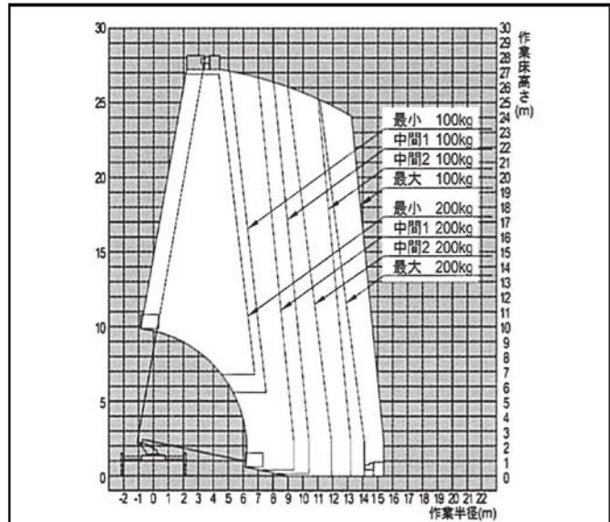
SK27A 作業範囲図
