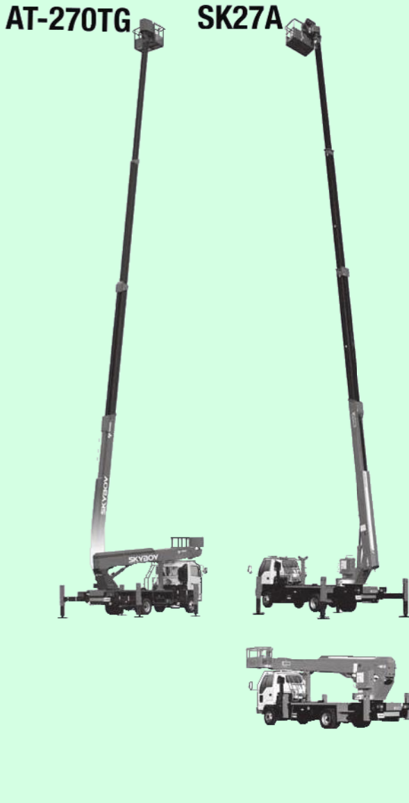
AT-270TG 作業範囲図
