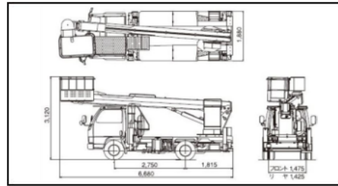
AT-170TG 作業範囲図
