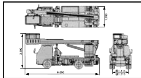
SK17A 外形寸法(mm)
