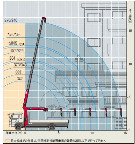
作業領域図
